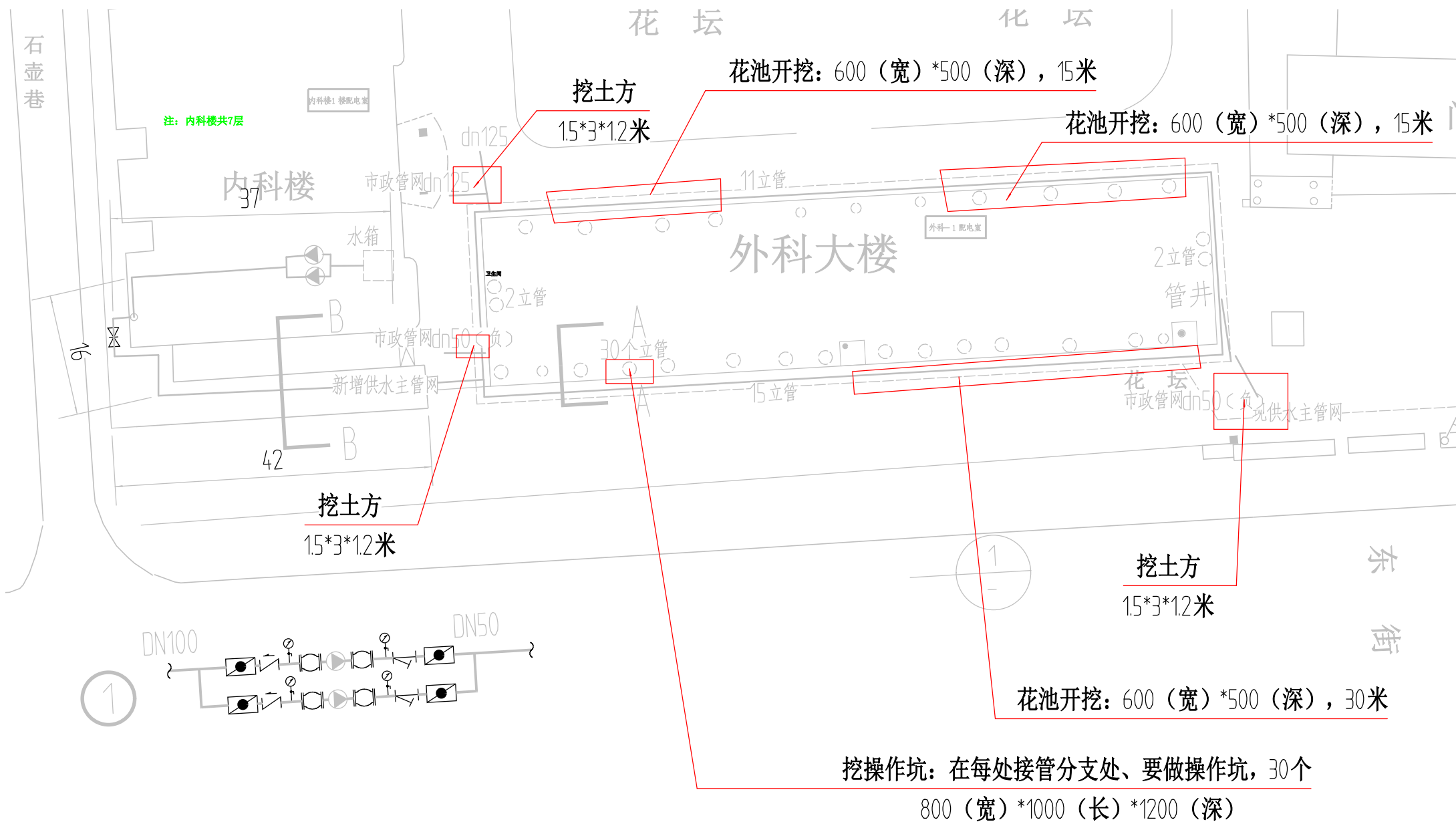
安装管道开挖地面位置示意图
